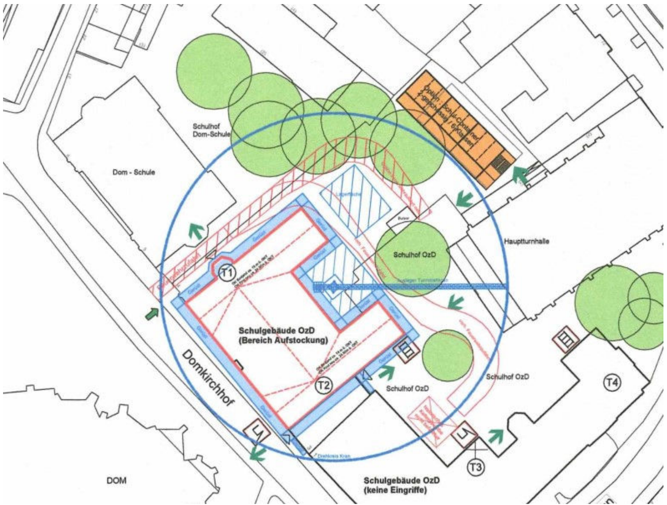
Lageplan + Baustelleneinrichtung
