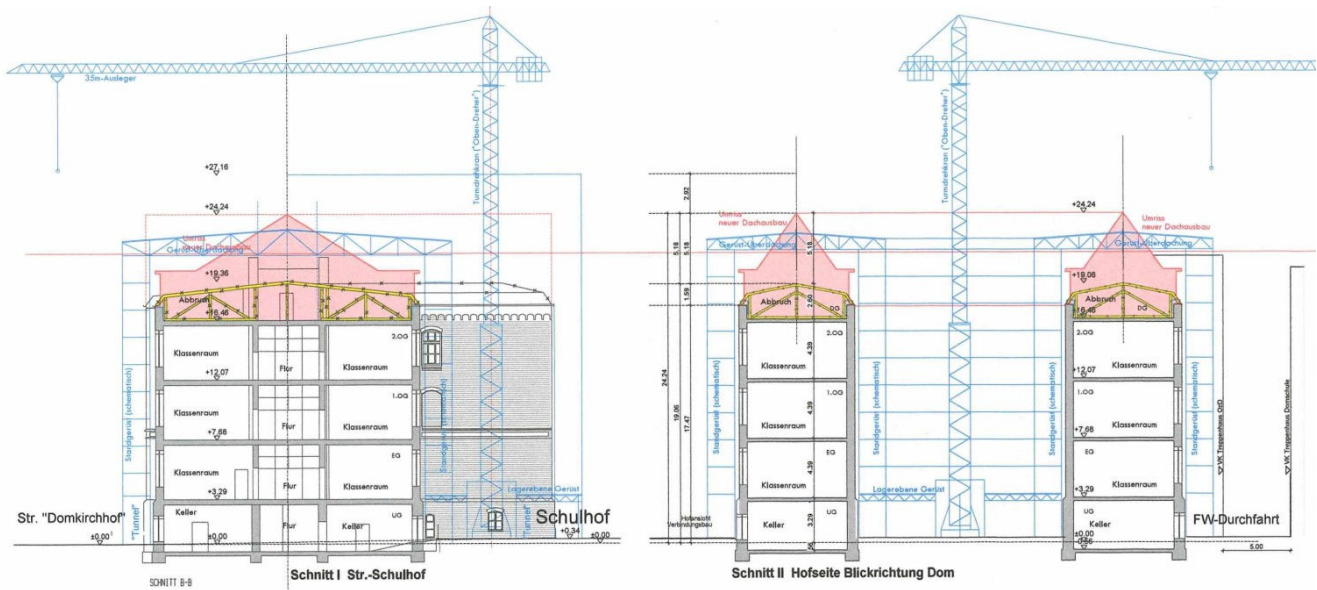
Schnitt + Baustelleneinrichtung
